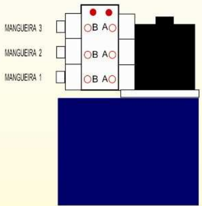
POSIÇÃO MANGUEIRAS 3 SAPATAS
